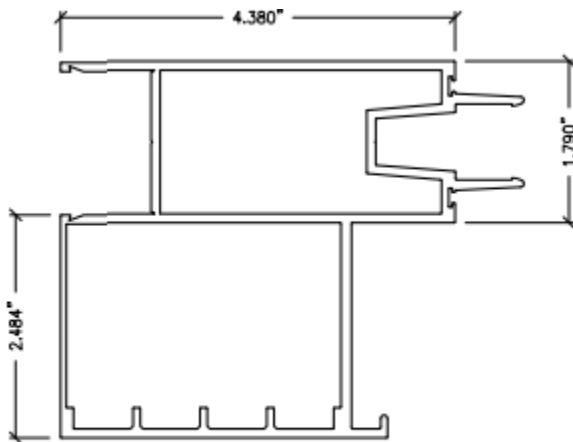
06 LOCK BUTT STILE (MALE) LIL-6
