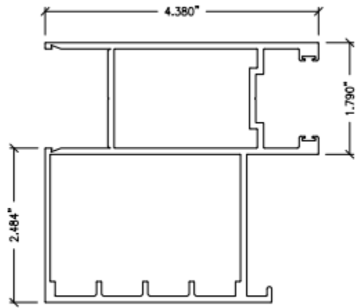
05 INTERLOCK BUTT STILE (FEMALE) LIL-5
