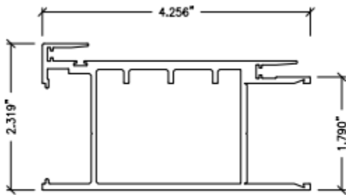
03 INTERLOCK STILE IL-3
