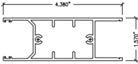
01 STD. DOOR RAIL DR-1
