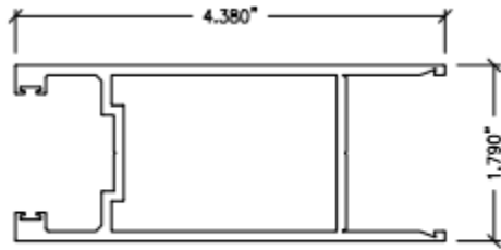
02 STD. DOOR STILE DS-2
